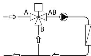
Valvola miscelatrice utilizzata in miscelazione
