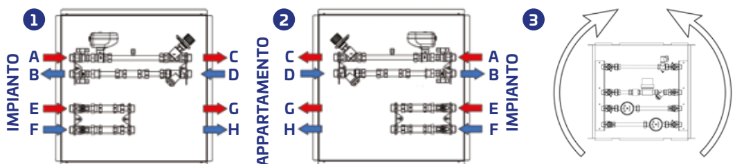
1- Modulo contabilizzazione montaggio lato sinistro
