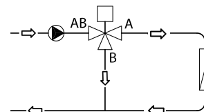
Valvola deviatrice utilizzata in deviazione
