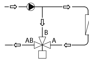
Valvola miscelatrice utilizzata in deviazione
